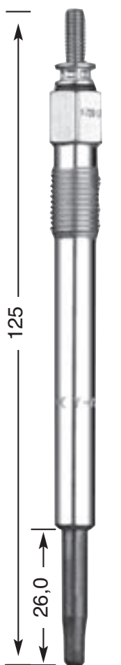
Y-729 U M 10 x 1.0 10 Hex 11,5 V DP 34
